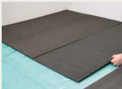
PANNEAUX ISOLANTS QUICKHEAT Panneaux isolants. 120 × 50 × 0,7 cm. 10 panneaux/lot. 0,6 m 2 /panneaux, 6 m 2 /lot. Épaisseur : 7 mm. Il est recommandé d'utiliser un pare-vapeur. Posez le film PE (PGUDLSCREEN34) sous les panneaux d'isolation QuickHeat et sur les éléments chauffants QuickHeat.
